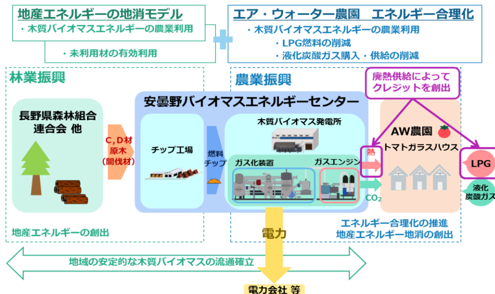
木質バイオマスによる地域エネルギー利用モデルの概要
