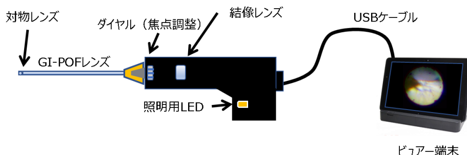
図2：Cellendo Scope システム構成
