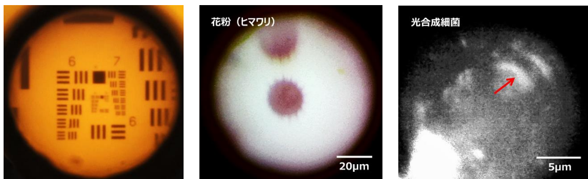
図1：左）GI-POF レンズと顕微鏡で撮影した解像度チャート、中）ヒマワリの花粉画像（約20μm）、右）北陸先端科学技術大学院大学 都英次郎教授提供 光合成細菌（ Rhodospseudomonas palustris 、体長約5μm）の極細内視鏡近赤外観察画像
